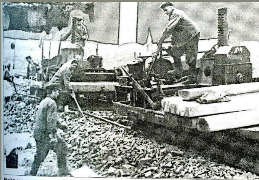
Идёт монтаж ж.д. путей на разрезе.
